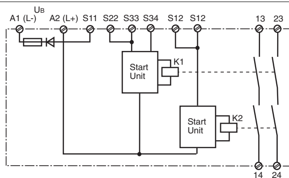
Fig. 2: PNOZ X5J Innenschaltbild/Internal Wiring Diagram/Schéma de principe
