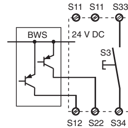
Fig. 6: nur bei PNOZ X5, PNOZ X5J: Eingangskreis einkanalig, manueller Start/ Only PNOZ X5, PNOZ X5J: Single-channel input circuit, manual reset/ Only PNOZ X5, PNOZ X5J uniquement: Commande par 1 canal, réarmement manuel
